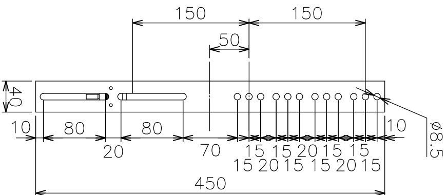
タッチメント穴位置図
