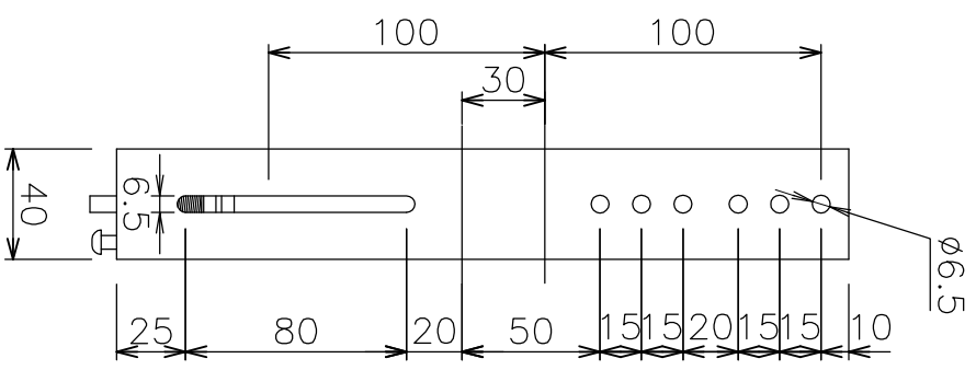
タッチメント穴位置図
